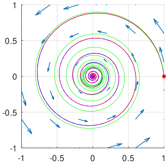
RK4 (m) / Euler (g) / Heun (r) / Exact (b)
